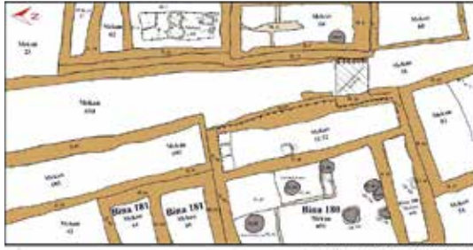
Kuzey Teras alanı genel planı (1/ 20 ölçek)
